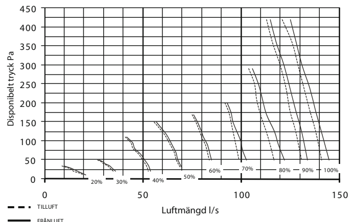
Pingvin eco XL till- och frånluftens kapacitetskurva med F5/F5 filter
