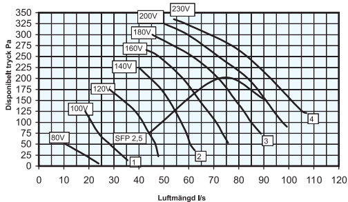
FENIX 120 FRÄNLUFT med EU5 planfilter Kapacitetskurva vid transformatorns olika spänningar 1, 2, 3 och 4 fabriksinställningar
